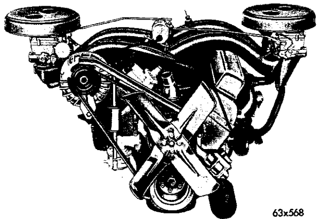
Fig. 58—C-300J Manifold
