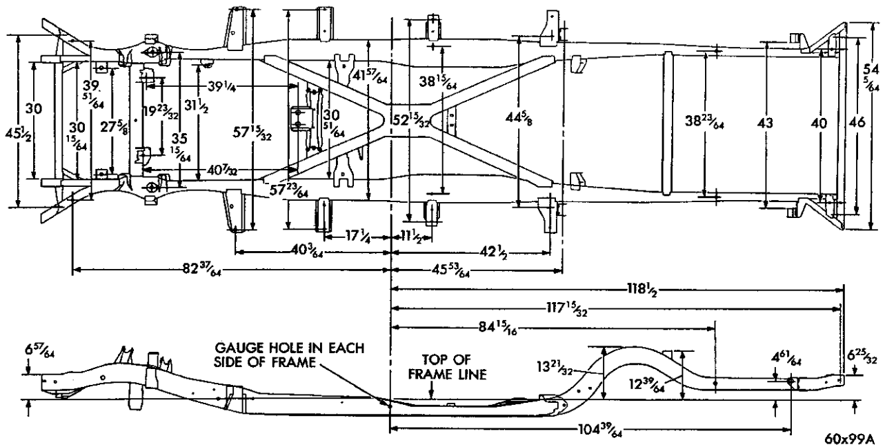
Fig. 2—Frame Dimensions (Imperial—Convertible)
