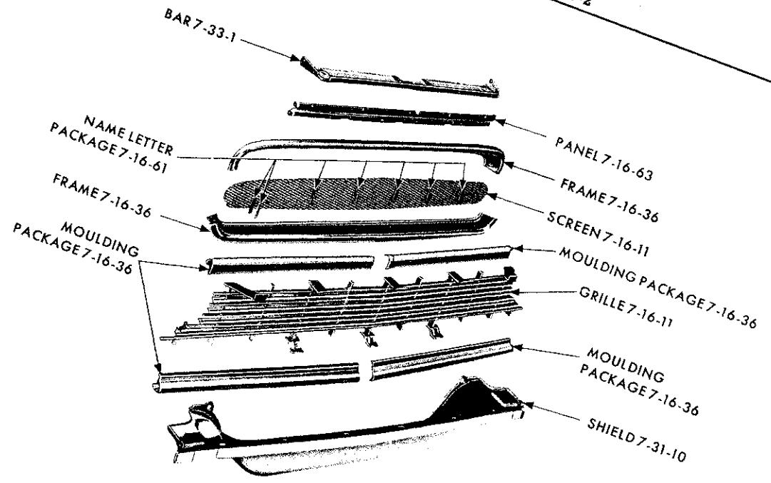
GRILLE - PLYMOUTH RP1-2
