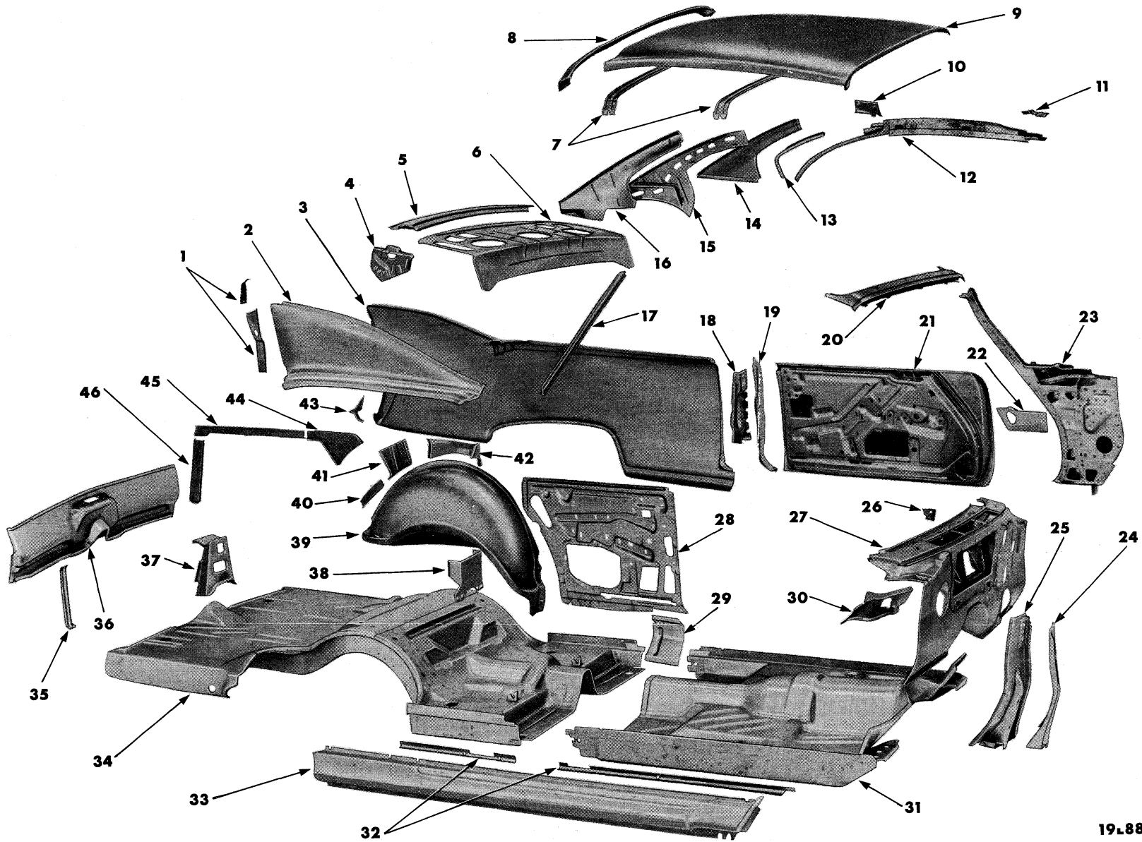
BODY - PLYMOUTH PP1-2 SPECIAL CLUB COUPE
