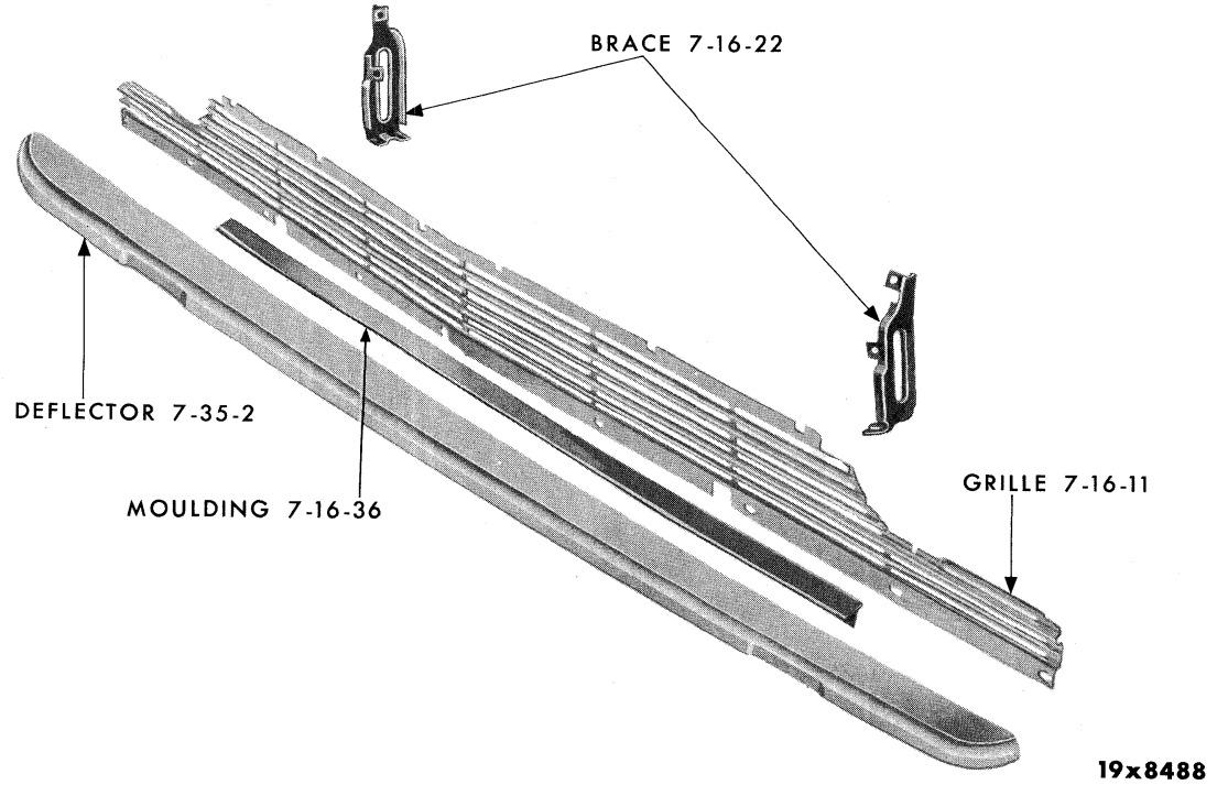
GRILLE - DESOTO MS1-2-3
