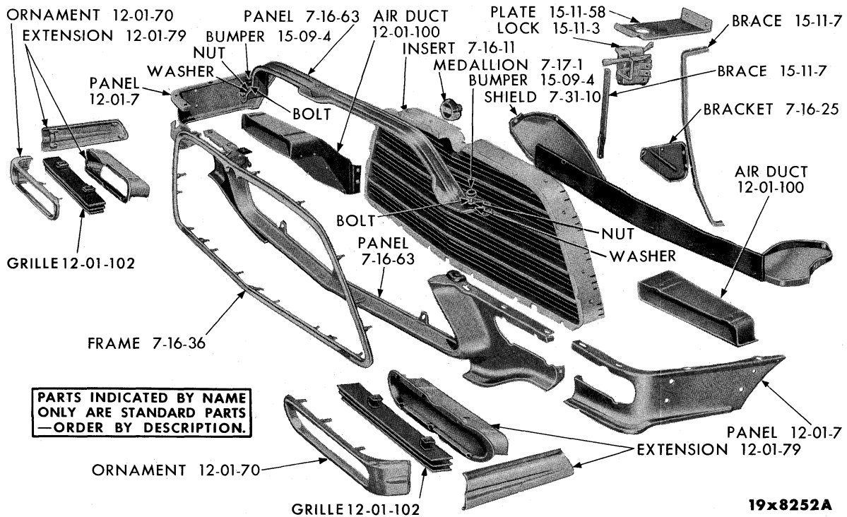
GRILLE - CHRYSLER MC300E
